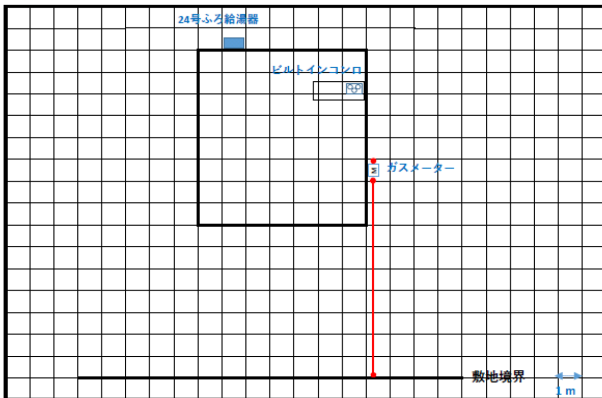
内管工事見積用平面図
